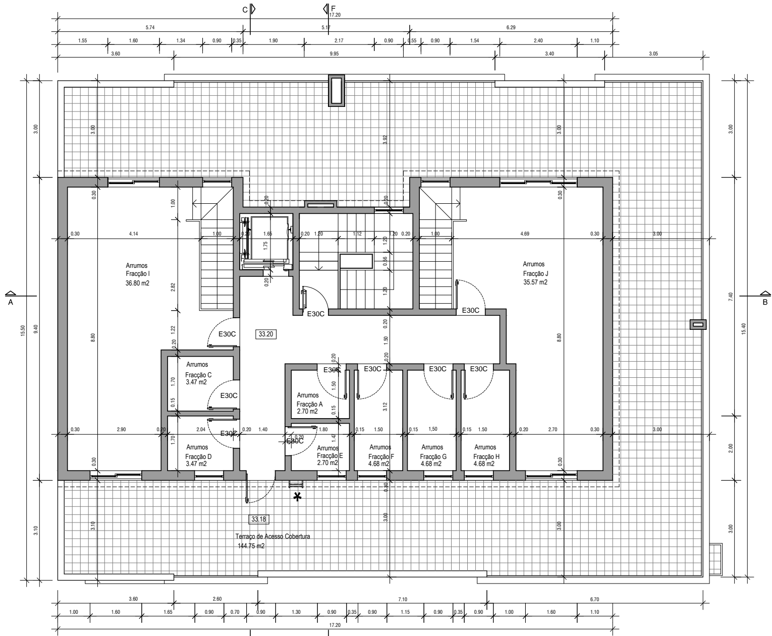
Planta do Piso do Sofão
