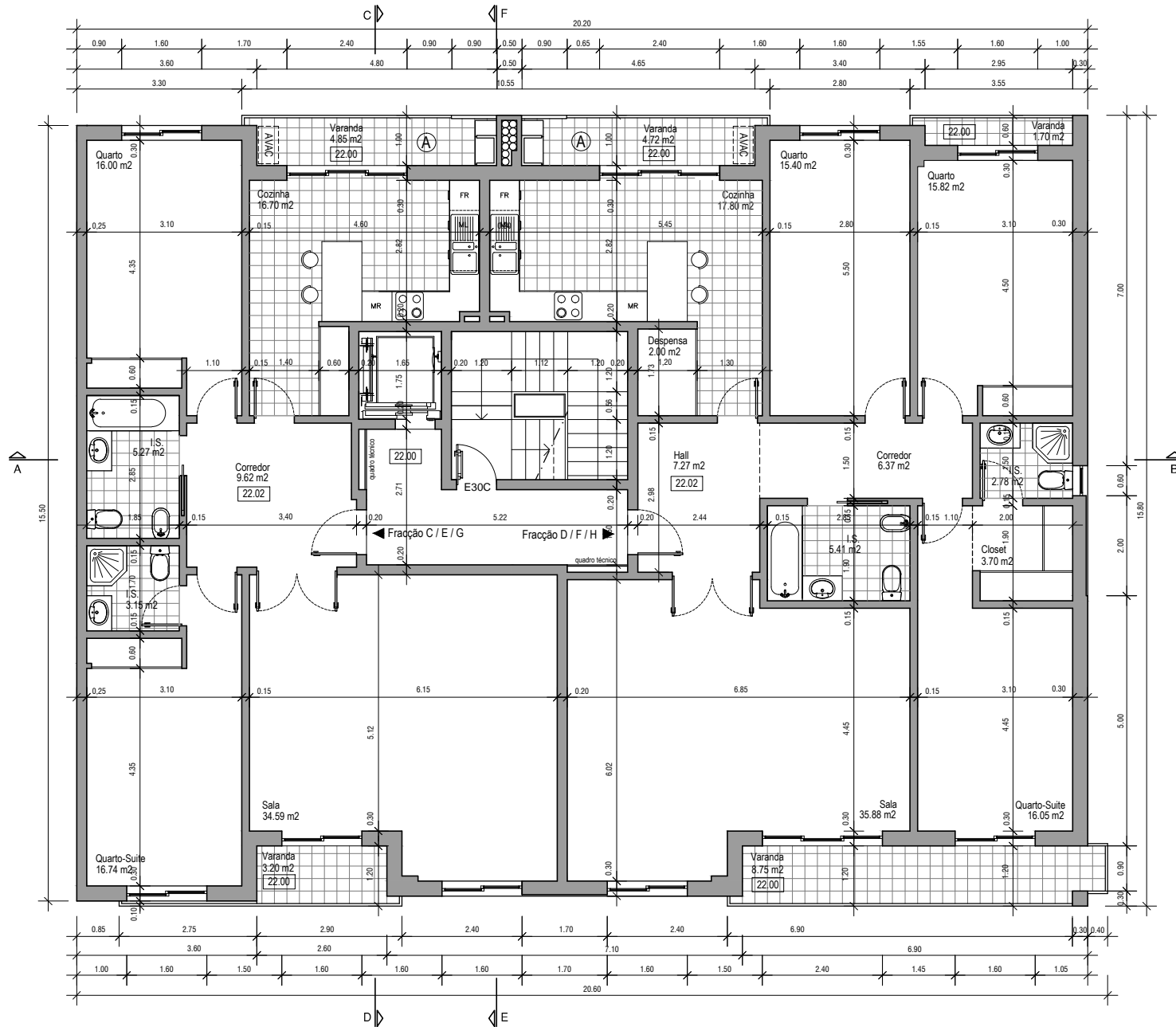
Planta do Piso 2 / 3 / 4
